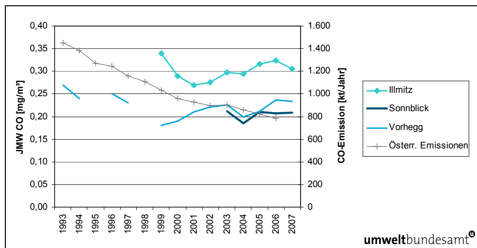
Abbildung 29: Jahresmittelwerte der CO-Konzentration sowie CO-Emissionen Österreichs, 1993 bis 2007 (in mg/m³).
