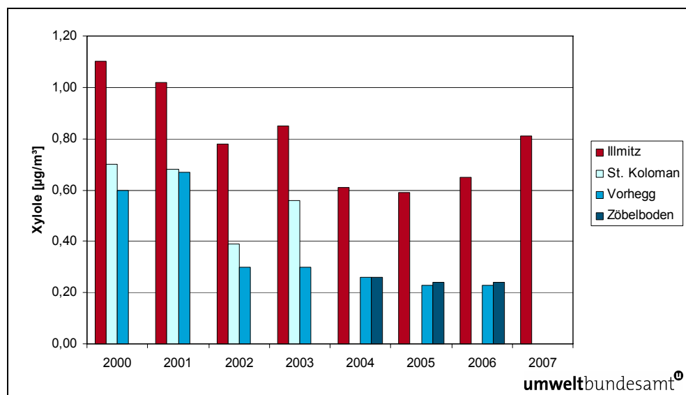
Abbildung 32: Verlauf der Xylolkonzentration, 2000 bis 2007 ( \mu\text{g}/\text{m}^3 ) (in Illmitz m-, p- und o-Xylol, in Vorhegg und Zöbelboden nur m-, p-Xylol, da o-Xylol meist unter der Nachweisgrenze lag).
