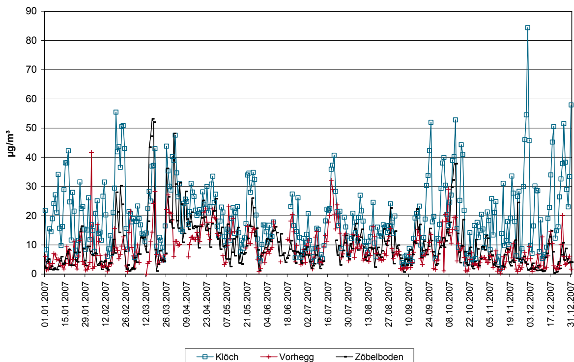
Abbildung 13: Tagesmittelwerte der PM 10 -Konzentration an den Messstellen Enzenkirchen, Illmitz und Pillersdorf (oben) sowie Klösch, Vorhegg und Zöbelboden (unten) im Jahr 2007 (in µg/m 3 ).
