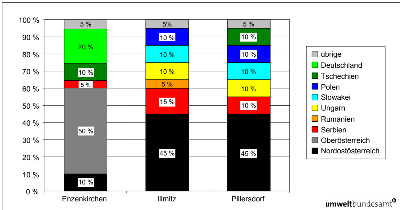
Abbildung 19: Abgeschätzte relative Anteile verschiedener Herkunftsregionen zur PM 10 -Belastung in Enzenkirchen, Illmitz und Pillersdorf, Tage über 45 \mu\text{g}/\text{m}^3 1999 bis 2007 (Herkunftsregionen mit Beiträgen über 5 %, gerundet auf 5 %; Übrige: Summe der Beiträge unter 5 %; Nordostösterreich: Wien, Niederösterreich, Nordburgenland).
