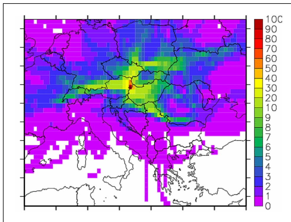
Abbildung 16: Häufigkeitsverteilung der Rückwärtstrajektorien für Illmitz, Winter 2002/03. Die Farbskalierung gibt die Häufigkeit in Prozent an, mit der die Rückwärtstrajektorien die einzelnen Rasterfelder überquert haben.
