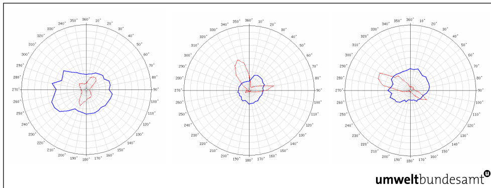
Abbildung 47: Schadstoffwindrosen für Klösch, Vorhegg und Zöbelboden (Wind Messturm; von links nach rechts), NO 2 , 2007.
