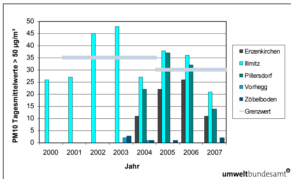
Abbildung 15: Anzahl der Tagesmittelwerte der PM10-Konzentration über 50 µg/m³, 2000–2007 (Enzenkirchen 2004 erst ab 29.1.).
