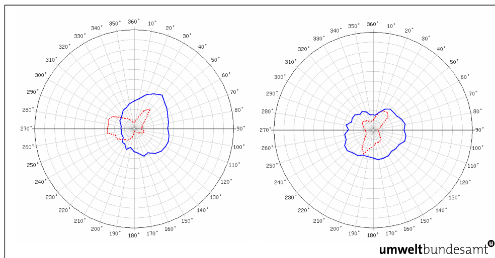
Abbildung 45: Schadstoffwindrosen für Pillersdorf (links) und Klösch (rechts), PM 10 , 2007, Rohdaten.
