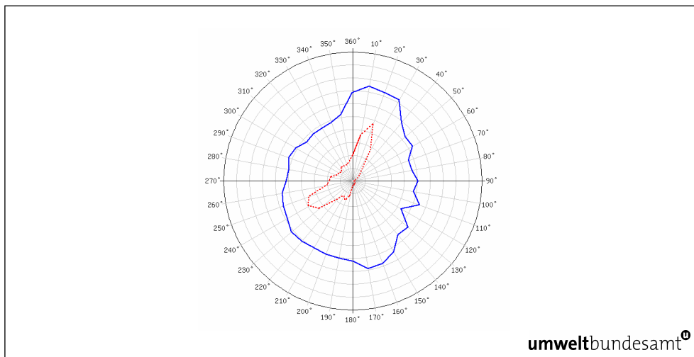
Abbildung 48: Schadstoffwindrose für den Sonnenblick, NO y , 2007 (Radius entspricht 2 ppb).
