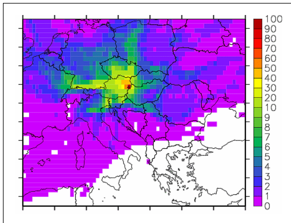
Abbildung 17: Häufigkeitsverteilung der Rückwärtstrajektorien für Illmitz, Winter 2005/06. Die Farbskalierung gibt die Häufigkeit in Prozent an, mit der die Rückwärtstrajektorien die einzelnen Rasterfelder überquert haben.
