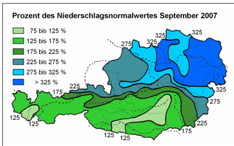
Abbildung 43: Abweichung der Monatssumme des Niederschlags im September 2007 vom mittleren Klimawert 1961–1990 (Quelle: ZAMG, www.zamg.ac.at ).
