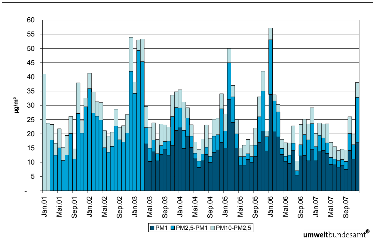
Abbildung 23: Monatsmittelwerte der Konzentration der Fraktionen PM1, PM2,5-PM1 sowie PM10-PM2,5 in Illmitz, 2001 bis 2007 (in \mu\text{g}/\text{m}^3 ).
