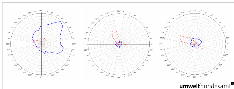
Abbildung 50: Schadstoffwindrosen für Pillersdorf, Vorhegg und Zöbelboden (Wind Messturm; von links nach rechts), \text{SO}_2 , 2007.
